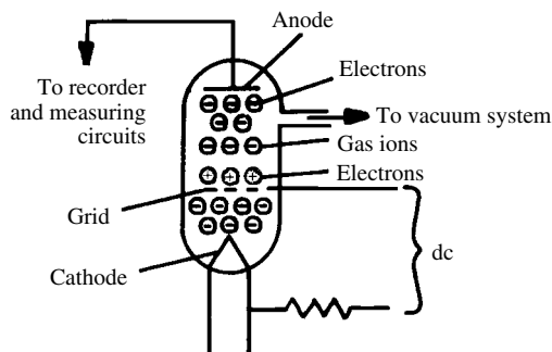
ionization gauge
