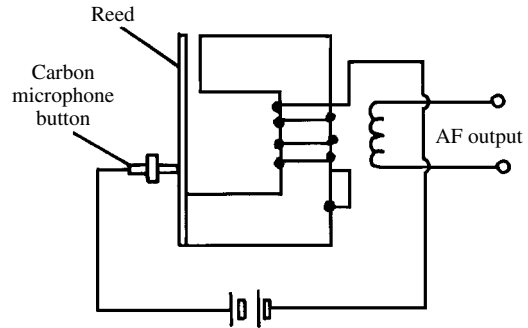
hummer
