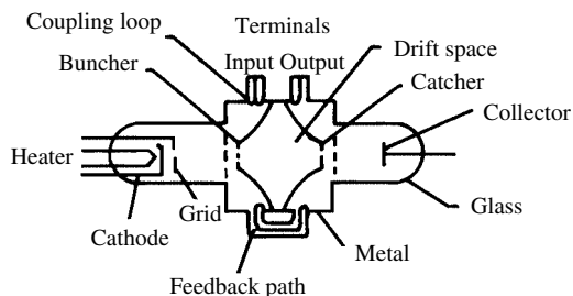
klystron
