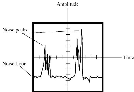
sferics
