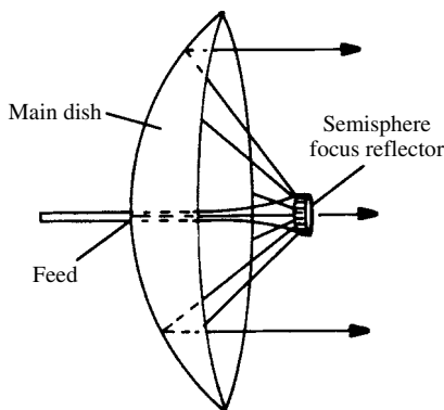
Cassegrain antenna
