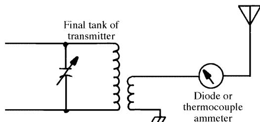
antenna ammeter
